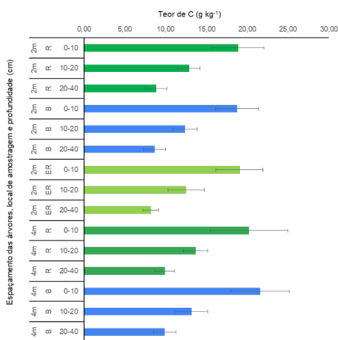
Figura 1. Teor médio \pm desvio-padrão de C ( \text{g kg}^{-1} ) em Argissolo Amarelo textura argilosa sob sistema integração pecuária-floresta, em Valença, RJ. Espaçamento das árvores dentro do renque (2 e 4m); R: renque de plantas de eucalipto; B: borda do renque, a 2 m do renque e ER: entre renque, cerca de 7-8 m do renque.
